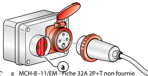
a MCH-8 -11/EM - Fiche 32A 2P+T non fournie b MCH-13/ET - Fiche 16A 3P+T non fournie
